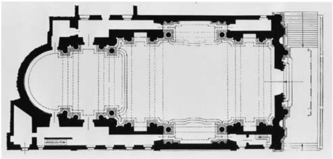
180. Mondovì, S. Francesco Saverio (Chiesa della Missione), Grundriss.
