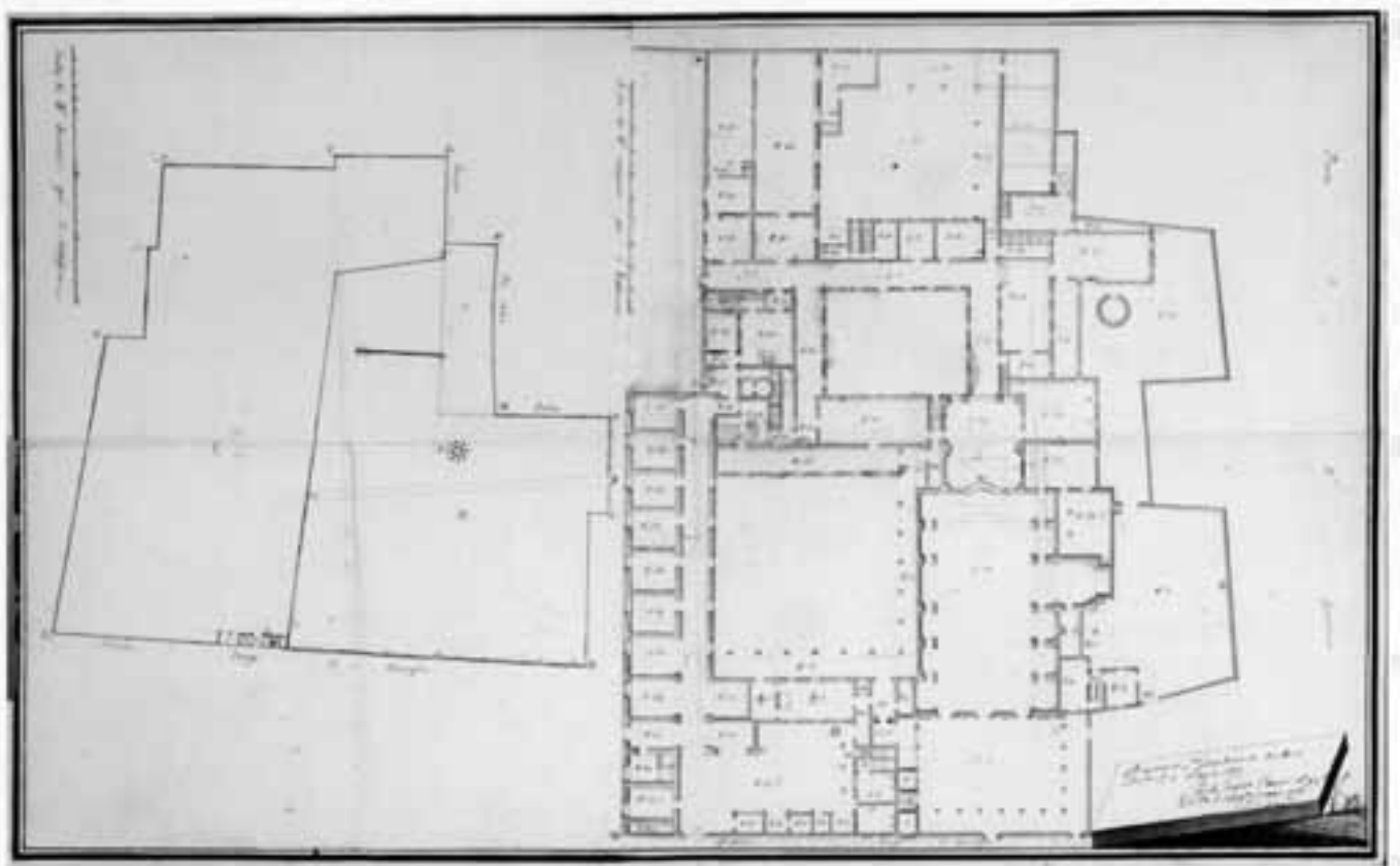
169. Mailand, Noviziatshaus, Plan Nr. 3.
